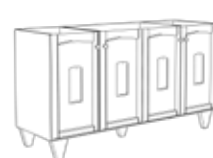
216 4 Larg. x Alt. x Prof. 1600 x 873 x 500mm
